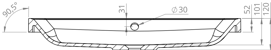
PRZEKRÓJ G-G SKALA 1 : 7
